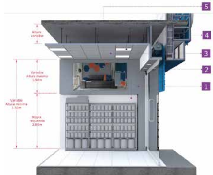
Detalle 2 Cajillo perimetral para Local con doble altura
