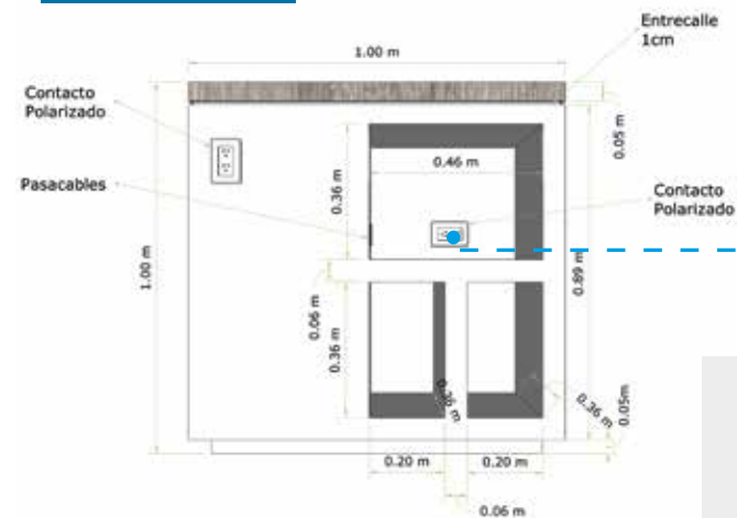
Alzado Lado 4
