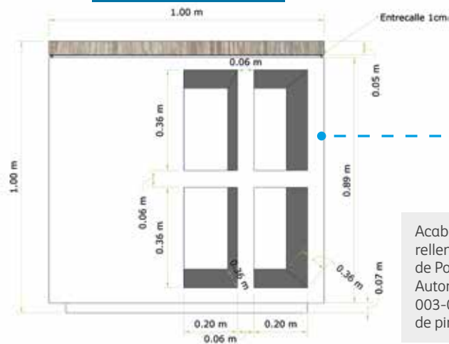
Alzado Lado 1,2,3
